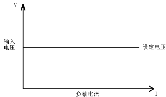
图3-2 恒电压模式
