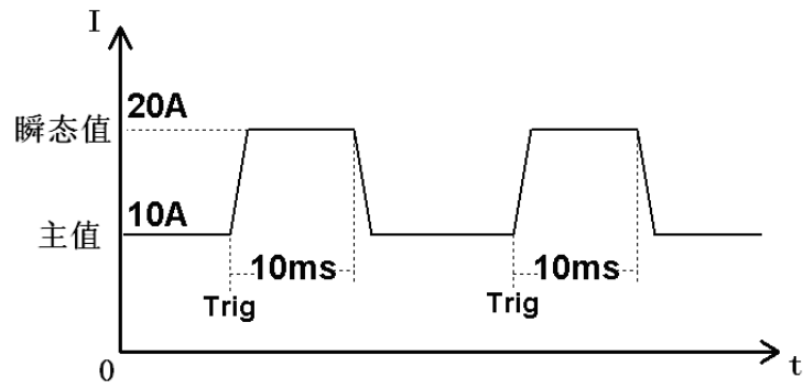
图3-6 脉冲方式
