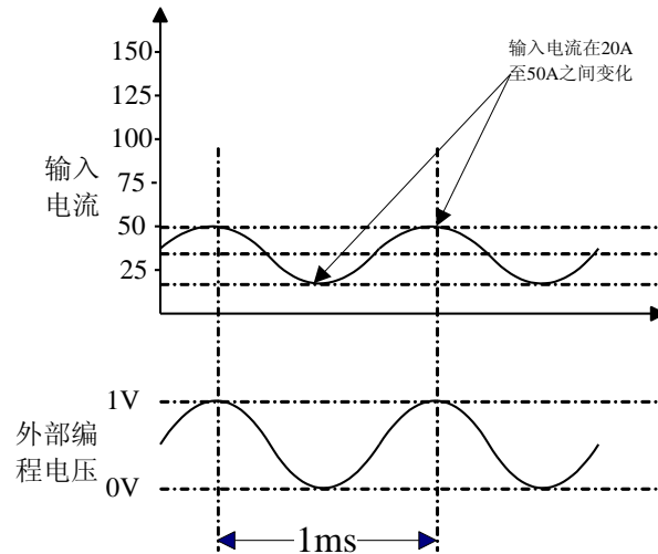
图 3-16 外部编程输入
