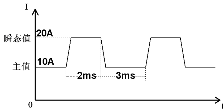
图3-5 连续方式
