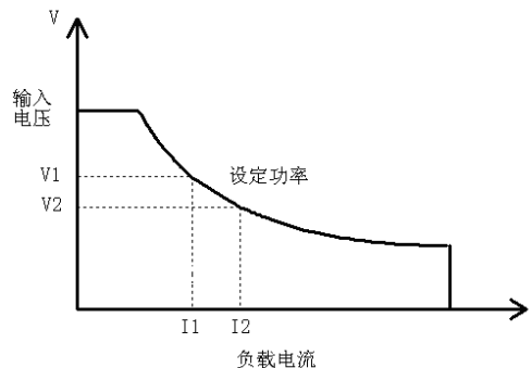
图3-4 恒功率模式
