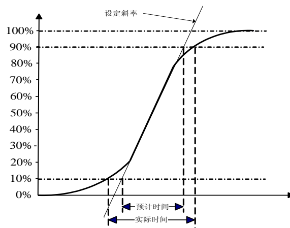
图 3-14 斜率与实际转换时间的关系
