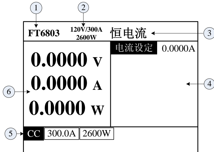
图 4-2 监视界面
