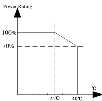
带载功率与操作温度间的关系
