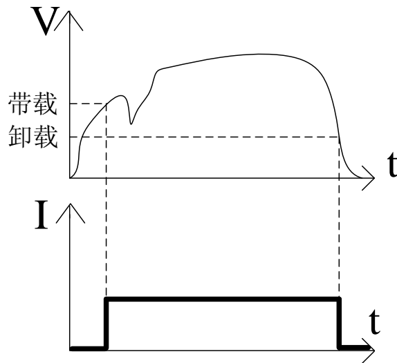
图 3-13 带载、卸载功能示意图
