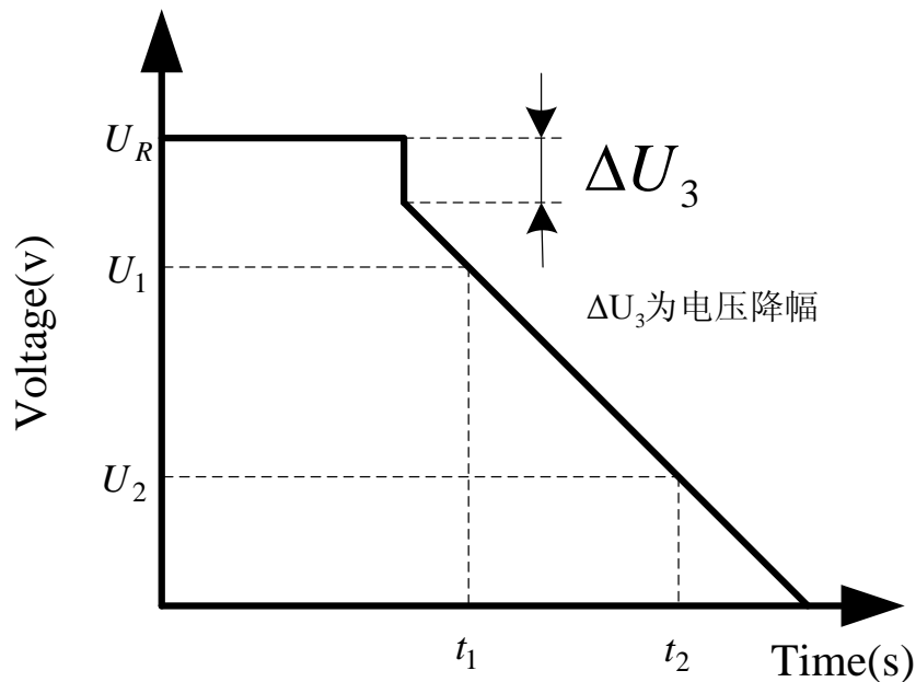
图 3-12 超级电容放电曲线图
