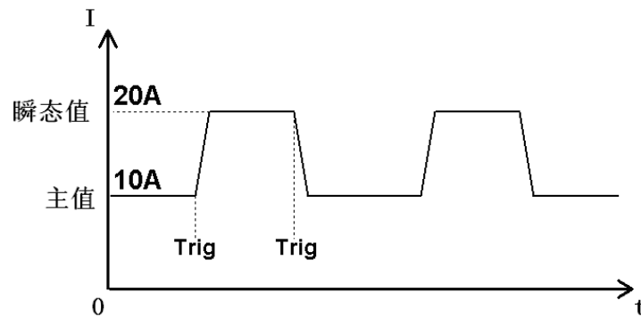
图3-7 翻转方式
