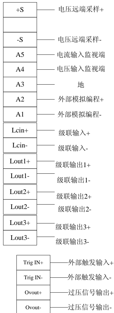
图 3-15 负载后面板控制、监视端子
