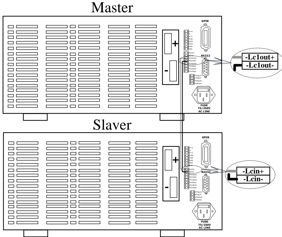
图 3-17 负载级联接线
