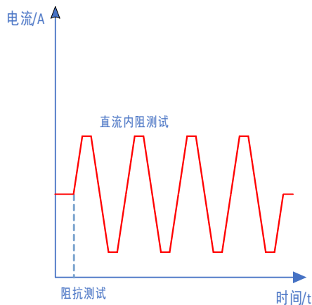
直流阻抗测试
